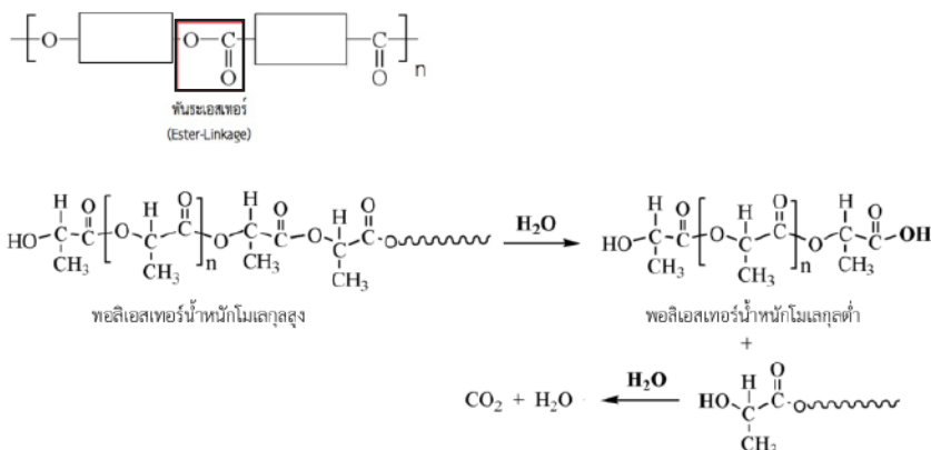
รูปที่ 3.1 โครงสร้างโมเลกุลจำลองของพอลิเอสเทอร์แสดงพันธะเอสเทอร์ และการย่อยสลายของตัวอย่างของพอลิเอสเทอร์ด้วยปฏิกิริยาไฮโดรไลซิส
